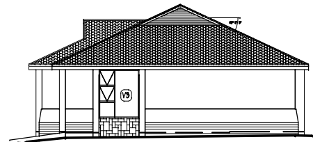
OOSAANSIG SKAAL 1:100
