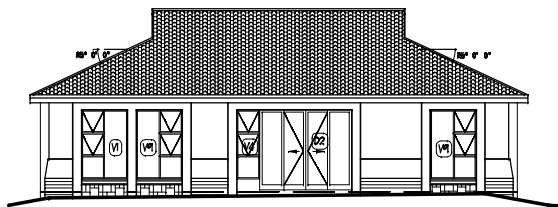
NOORDAANSIG SKAAL 1:100
