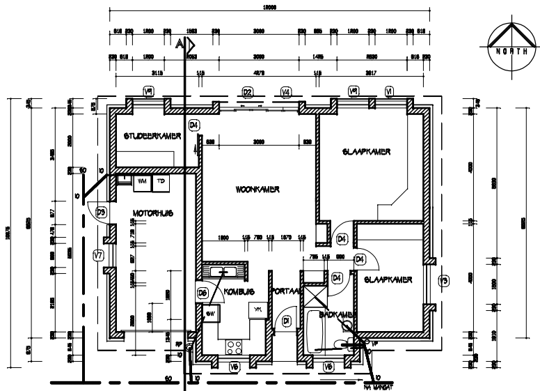
GRONDVOERPLAN SKAAL 1:100
